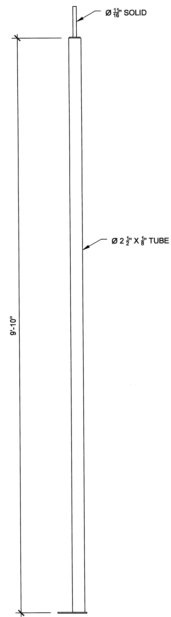
6 DINING TENT SIDE POLE SCALE: 1" = 1'-0"
