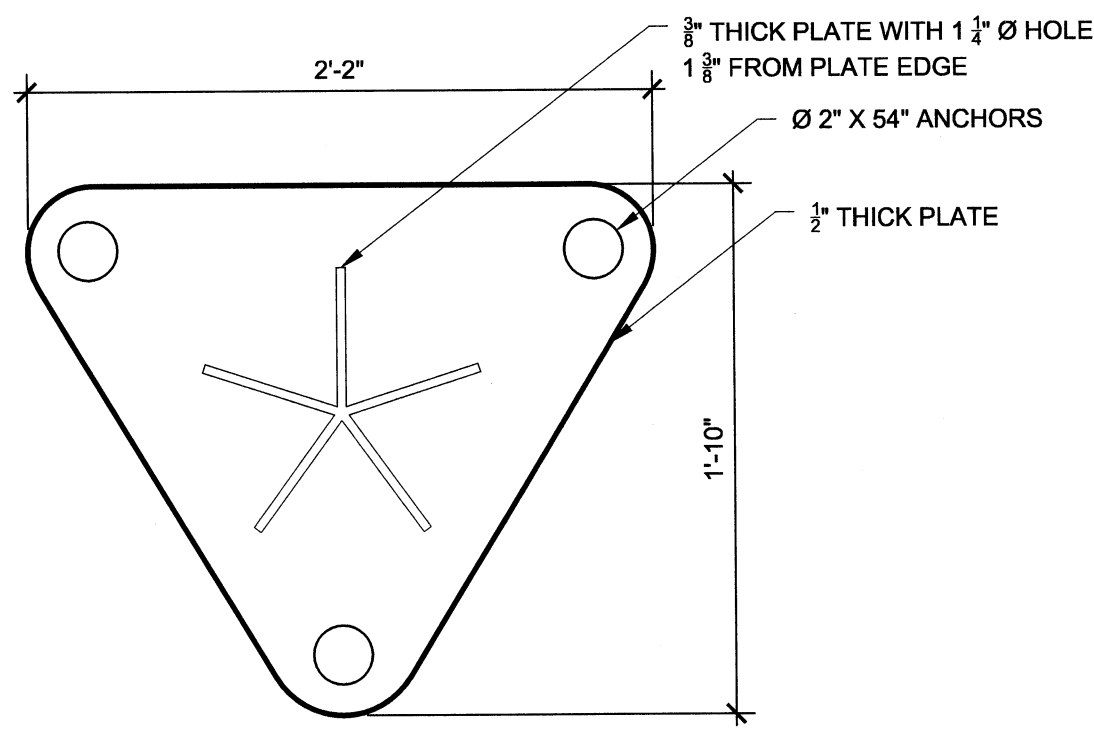
3 ANCHOR PLATE SCALE: 1 1/2" = 1'-0"
