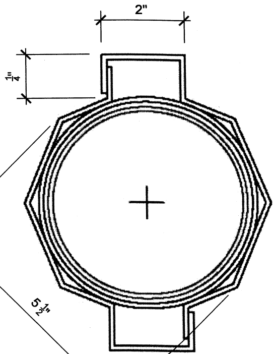
10 SECTION A-A SCALE: 1" = 1'-0"
