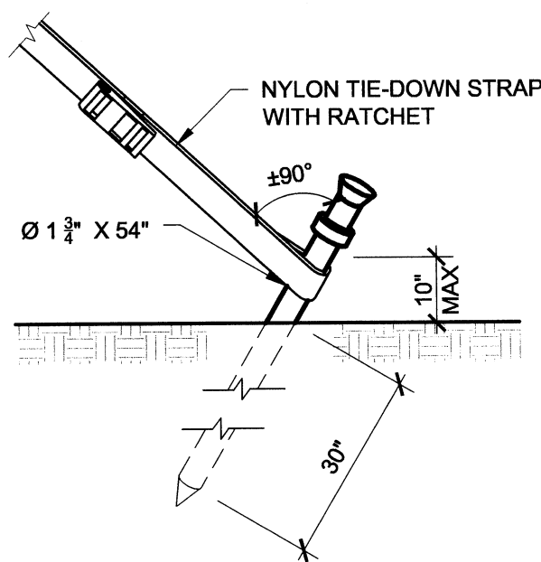
2 ANCHOR STAKE SCALE: 1" = 1'-0"
