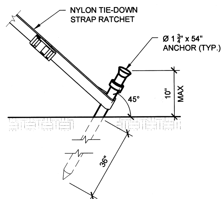
5 ANCHOR STAKE SCALE: 1" = 1'-0"
