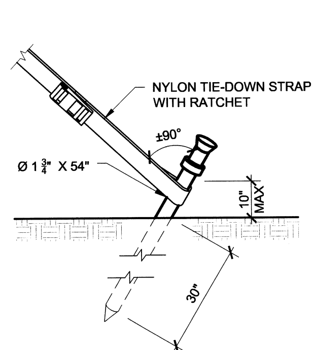
2 ANCHOR STAKE SCALE: 1" = 1'-0"
