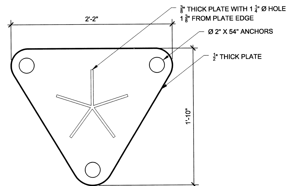
3 ANCHOR PLATE SCALE: 1 1/2" = 1'-0"
