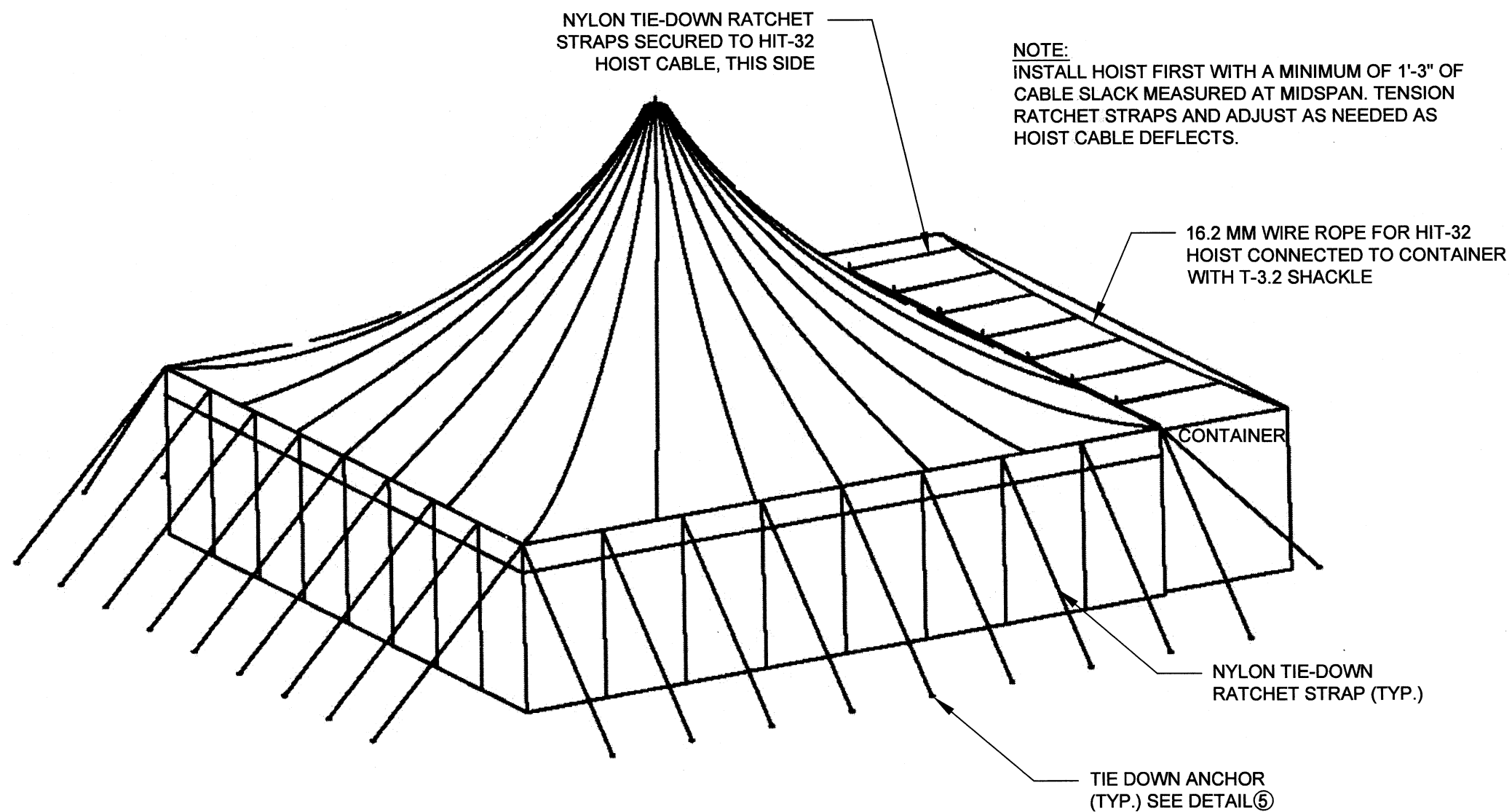
4 DINING TENT ISOMETRIC VIEW SCALE: N.T.S.
