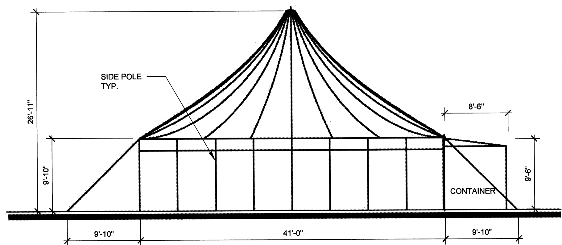
2 DINING TENT ELEVATION SCALE: 1/8" = 1'-0"
